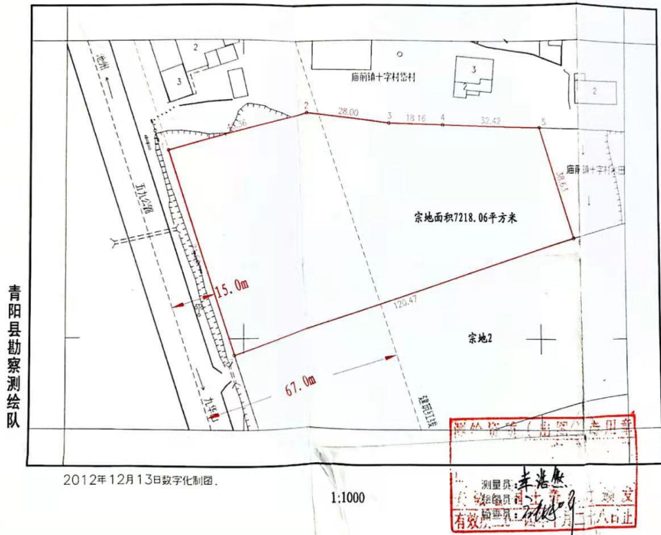
安徽拓富置业投资有限公司 (大九华旅游用品展示园1) 宗地图
